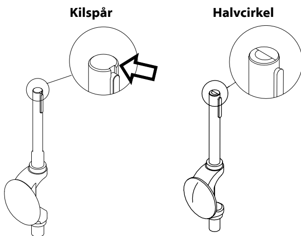
Fig.5-4 Markering för kulsegmentets läge i ventilen.
