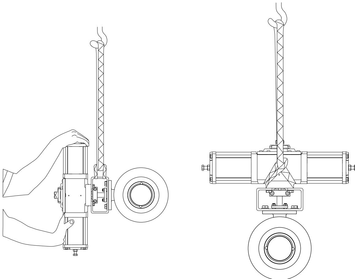
Fig.5-1 Lyftinstruktion
