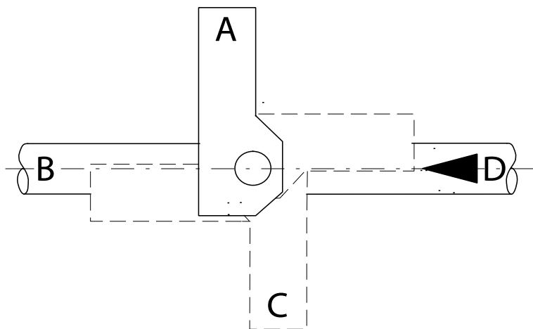
Fig.5-6 Ställdonets monteringslägen
