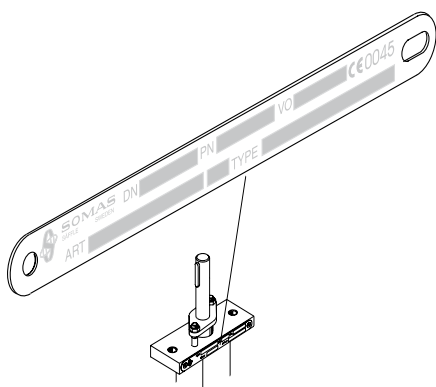
Fig.6-1 Dataskylt
