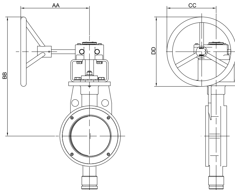
Поворотная заслонка тип VSS PN 40/ Class 300 с рычагом управления
