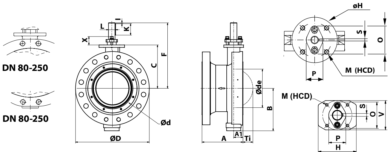
Поворотная заслонка тип VSSF PN 40/ Class 300
