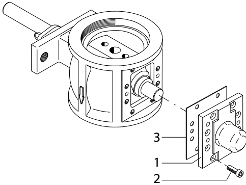
Şekil 6-3 Contanın deęiřtirilmesi
