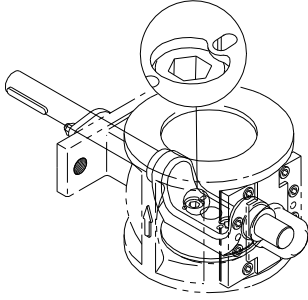
Fig.6-24 DN 40-250 civataları kilitleyin
