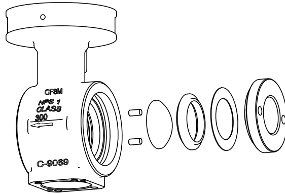
Fig.6-11 Yatağın değiştirilmesi DN 25-50
