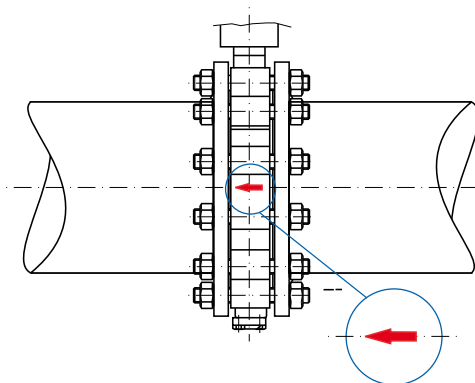
Fig. 5-2 Riferimento della direzione di flusso preferibile
