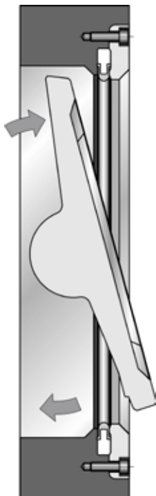
Fig.3-1 Funzionamento della valvola
