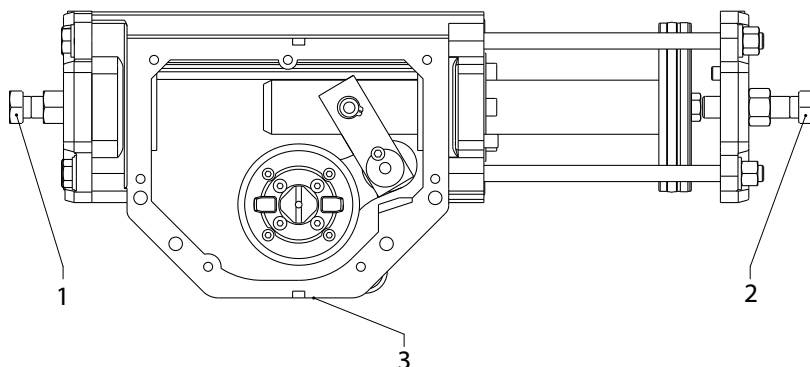
1 Posizione "aperta" del bullone terminale 2 Posizione "chiusa" del bullone terminale 3 Targhetta identificativa
