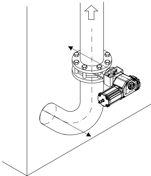
Fig.5-3 Inmontering nära rörkrök
