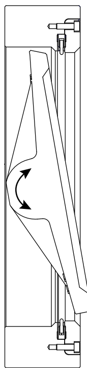
Fig.3-2 Ventilfunktion VSS Fire safe
