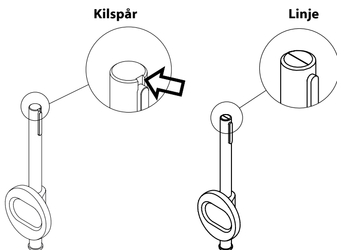
Fig.5-8 Markering av spjällets läge i ventilen.
