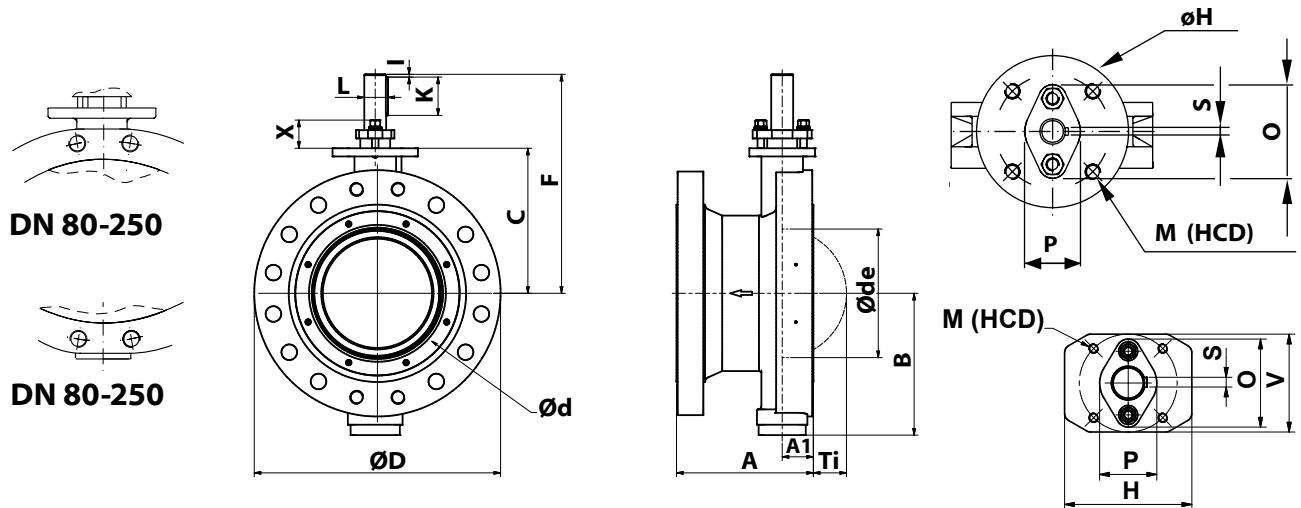
Butterfly valve type VSSF PN 40 /Class 300
