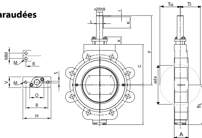
Vanne papillon type MTVL
