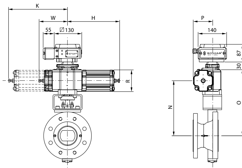
Поворотная заслонка тип MTFV с приводом тип A-DA
