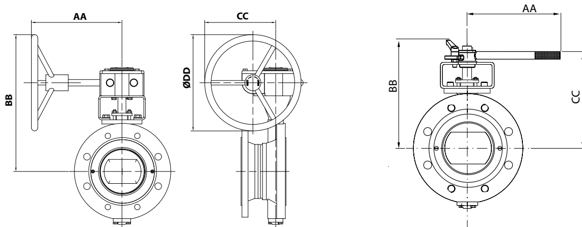
Поворотная заслонка тип MTVF с рычагом управления
